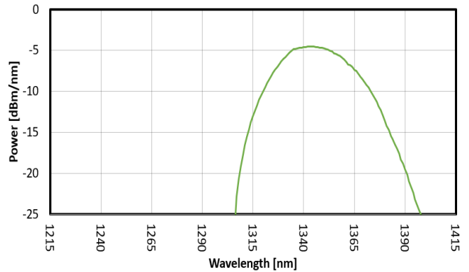
FIG. 2: SLED 1 SPECTRUM
