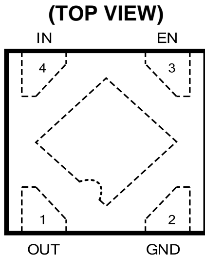
UTDFN-1x1-4
